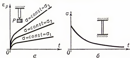
Рис. 2. а — кривые ползучести ε p металлов при различных нагрузках; б — кривые релаксации напряжения σ при постоянной деформации.
